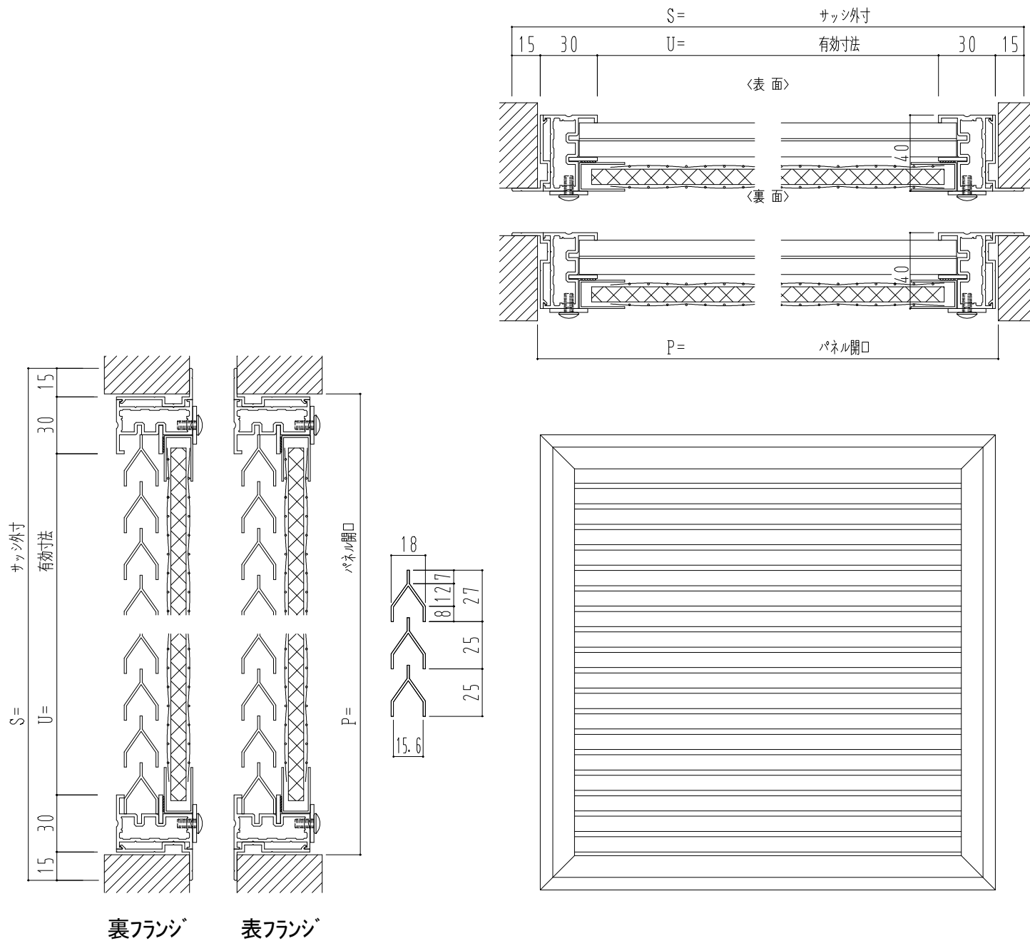
化粧アングル
