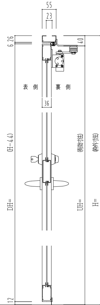
スレコ®長さ調整機能付 (12~20mm)
